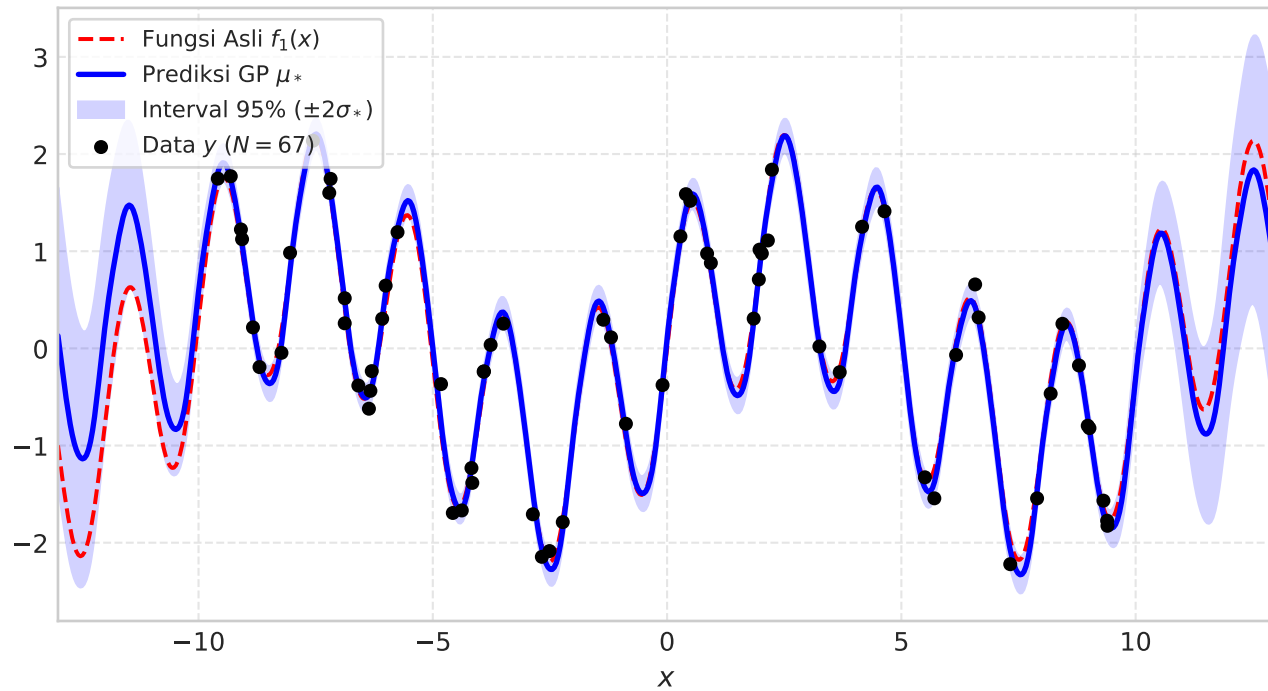
(c) Penjumlahan: k_{\text{Lin}} + k_{\text{Per}}
